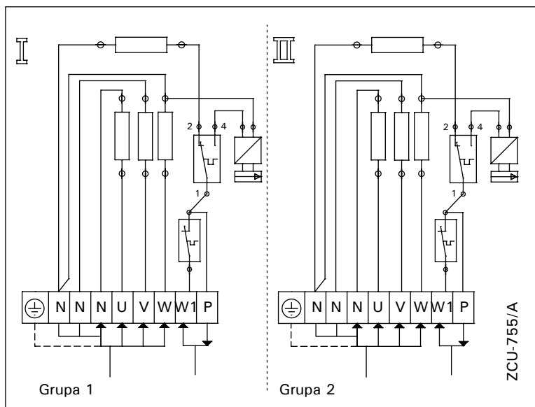
Rys. 9. Podłączenie elektryczne
